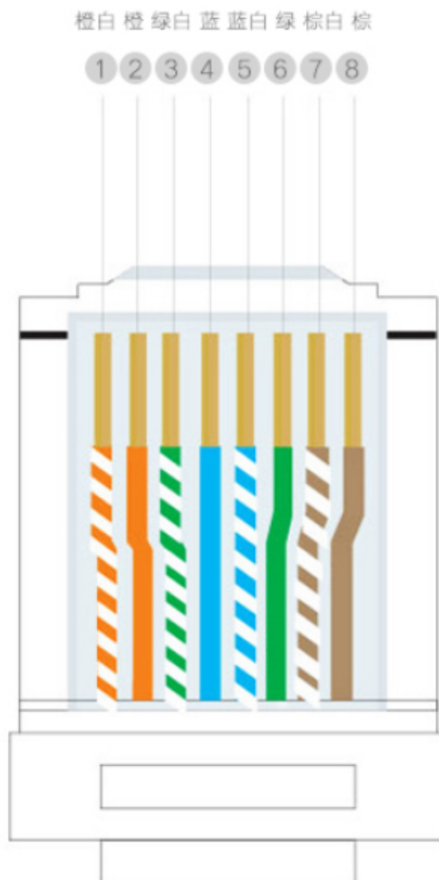
T568B标准:
