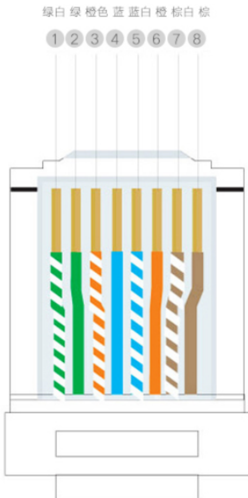
T568A标准:
